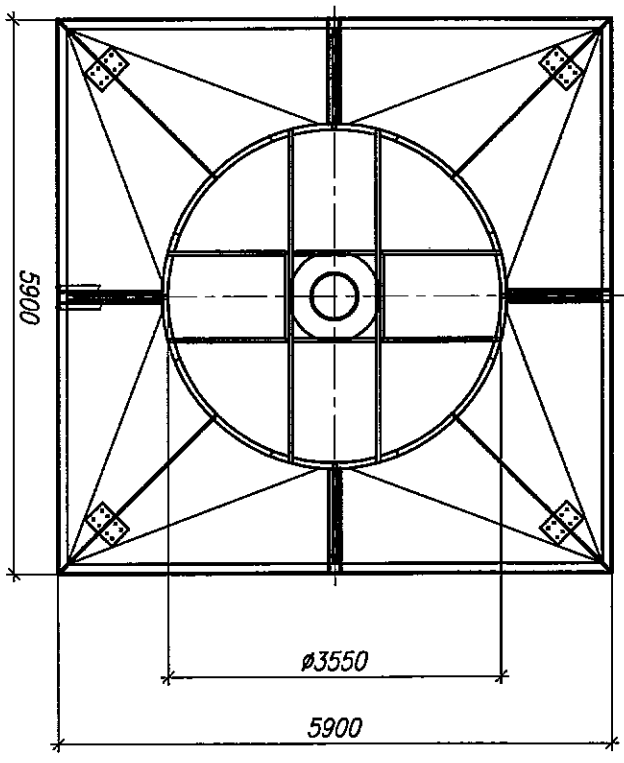
Draufsicht PLAN VIEW
